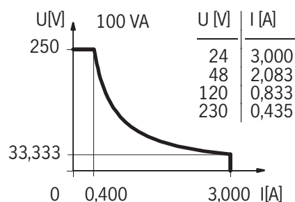
Schaltleistungsdiagramm
