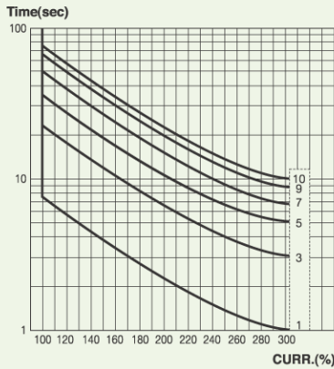
EOCR-SP1 반한시 특성곡선
