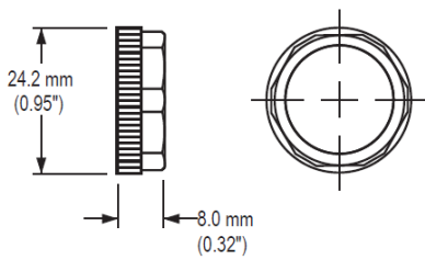
M18 x 1 Jam Nut
