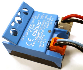
connecteur/connector WAGO 734-serie
